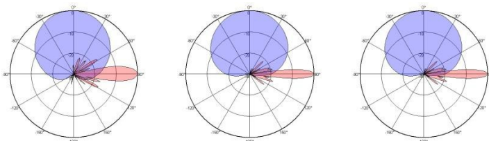
698~960MHz
